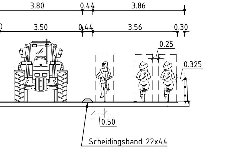
Profiel om-en-om-regeling viaduct A15
