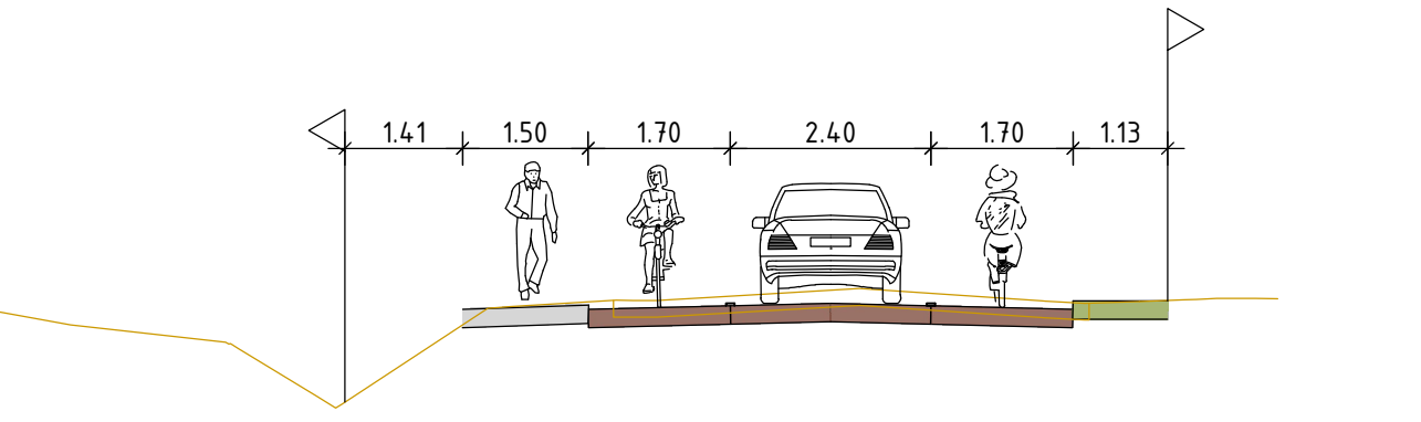
Normaalprofiel binnen bebouwde kom
