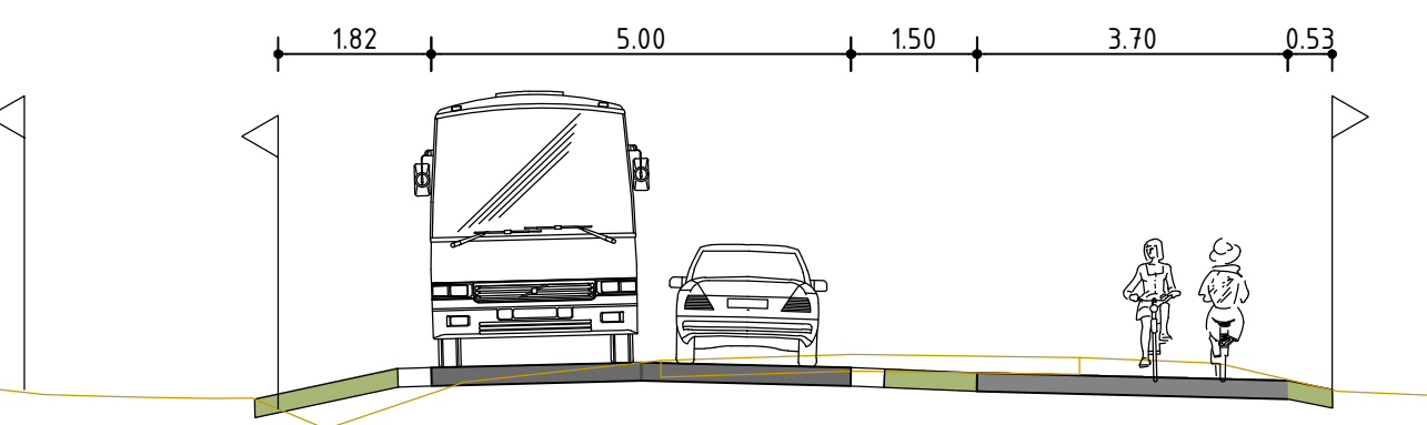
Normaalprofiel buiten bebouwde kom
